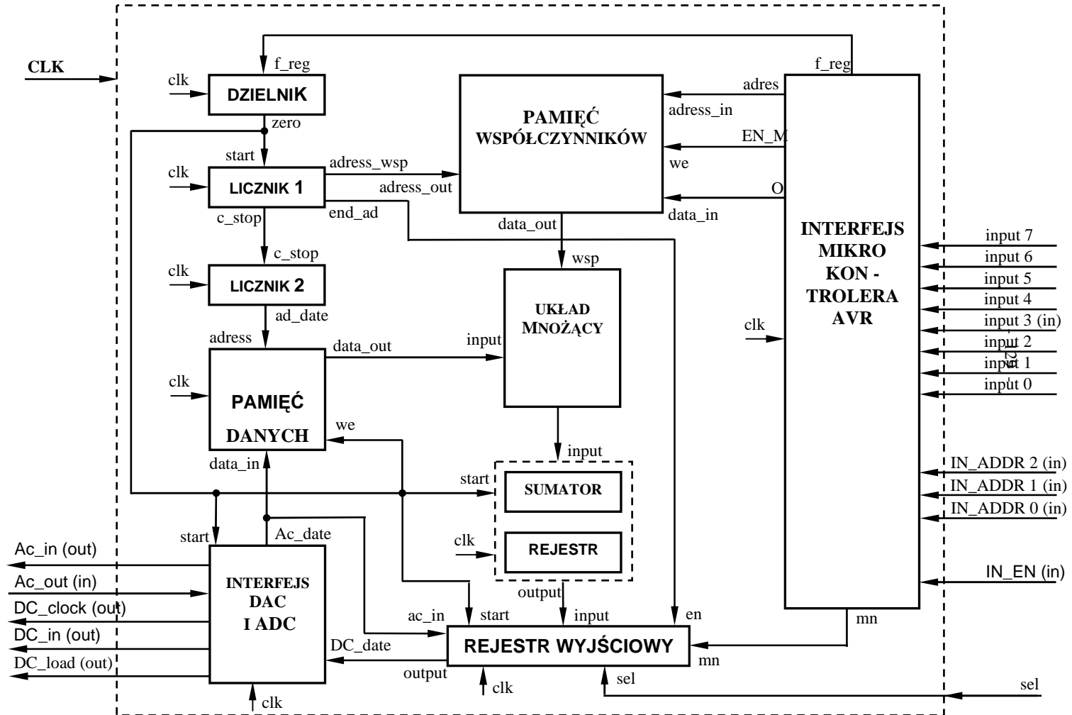
Rys.2. Schemat blokowy zaimplementowanego filtru [1].
