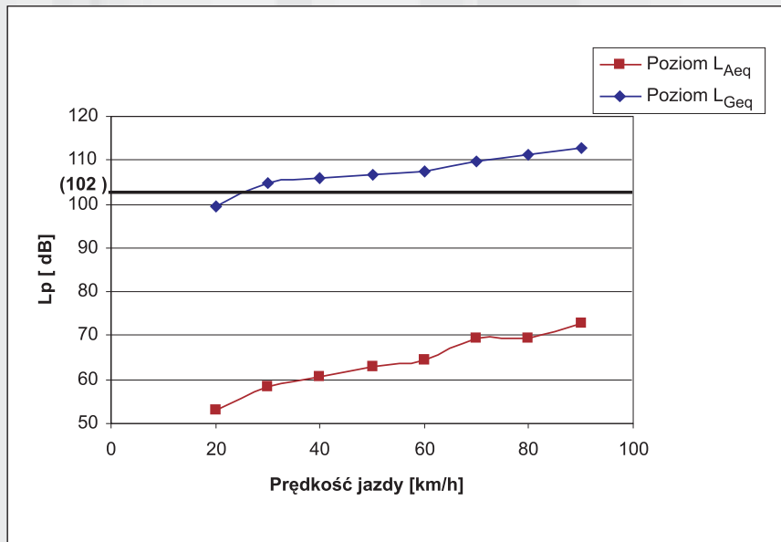
Rys. 1. Równoważny poziomu dźwięku A i G w zależności od prędkości jazdy na stanowisku pracy kierowcy autobusu miejskiego (pojazd kategorii M3/1)
