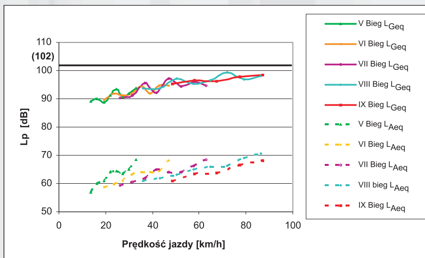
Rys. 2. Równoważny poziomu dźwięku A i G w zależności od prędkości jazdy na stanowisku pracy kierowcy ciężkiego samochodu ciężarowego (pojazd kategorii N3)
