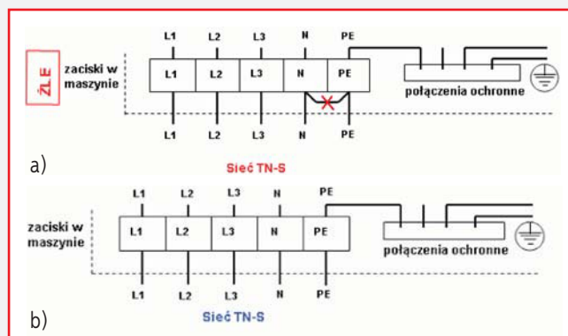
Rys. 2. Przykład zacisków maszyny w sieci TN-S: a) podłączenie nieprawidłowe; b) podłączenie prawidłowe
