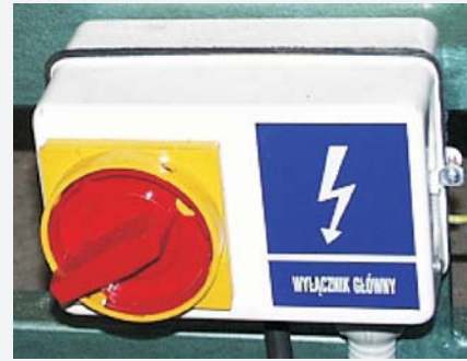
Fot. 10. Prawidłowy rozłącznik główny maszyny Photo 10. A proper machinery main switch
