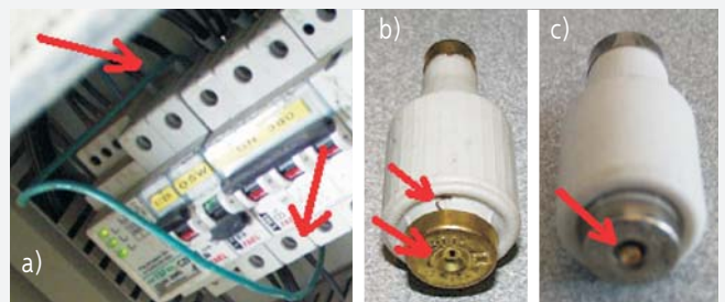
Fot. 8. Przykłady bezpieczników: a) zbrocznikowy wyłącznik nadprądowy przez połączenie przewodem zielonym jego zacisków; b) bezpiecznik „watowany”; c) nie-przepalony bezpiecznik
