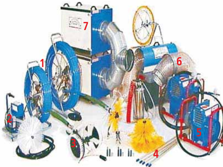
Rys. 1. Zestaw urządzeń do czyszczenia i dezynfekcji przewodów wentylacyjnych: 1 – urządzenia czyszczące pneumatycznie, 2 – małe urządzenia czyszczące, 3 – zestaw szczotek do różnego rodzaju kanałów, 4 – skrobaczki do tłuszczu, 5 – urządzenia odsysające, 6 – przewód do odprowadzania powietrza, 7 – zestaw filtrujący [2]
