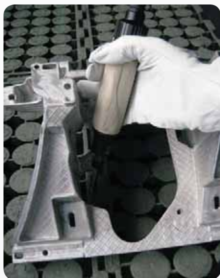
Fot. 1. Gradowanie w rękawicy roboczej Photo 1. Deburring in working glove
