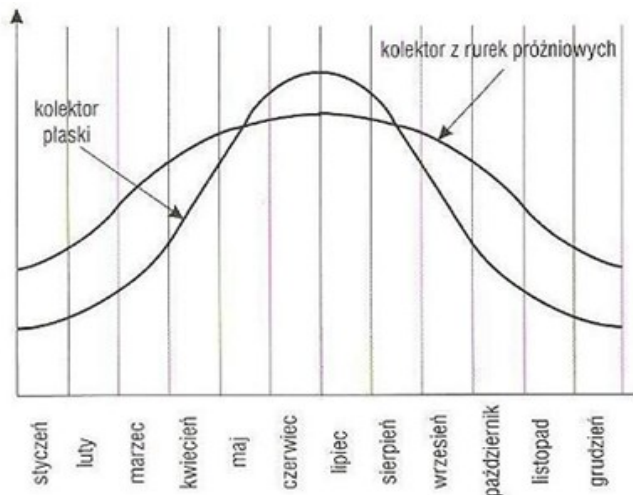
Rys. 1. Porównanie wydajności cieplnej kolektora płaskiego i próżniowo-rurowego [6]
