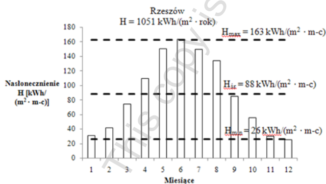
Rys. 2. Rozkład energii słonecznej docierającej do powierzchni Ziemi dla Rzeszowa
