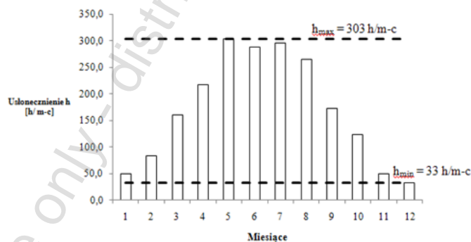
Rys. 3. Rozkład usłonecznienia w ciągu roku w Rzeszowie, dla J > 200 \text{ W}/\text{m}^2
