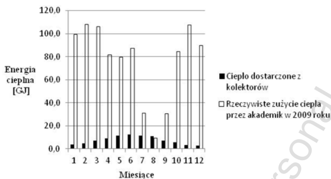
Rys. 4. Porównanie teoretycznej energii uzyskanej z kolektorów słonecznych z rzeczywistym zapotrzebowaniem na ciepło z 2009 roku
