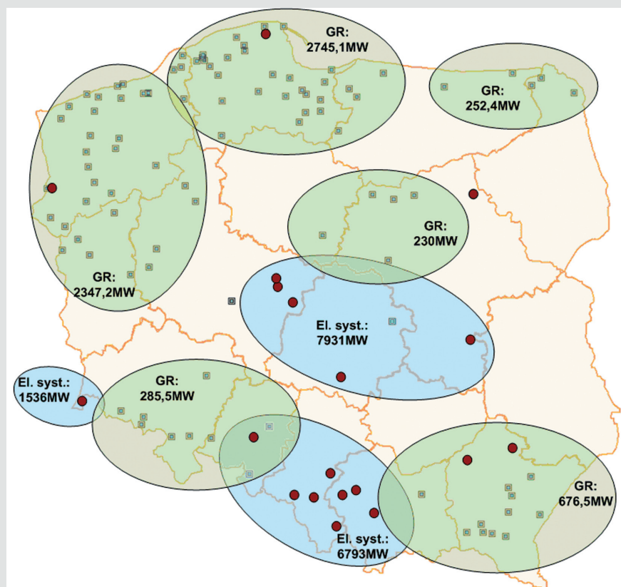
Rys. 3. Podział KSE na obszary o skoncentrowanym wytwarzaniu
