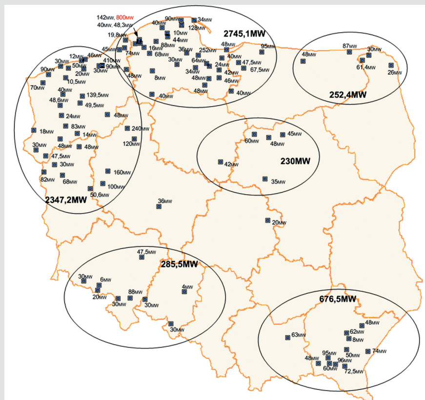
Rys. 2. Rozmieszczenie oraz moce znamionowe farm wiatrowych pracujących w KSE 3
