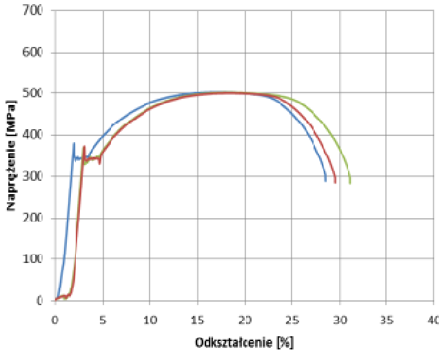
Rys. 3. Krzywe rozciągania w statycznej próbie dla próbek: a) w stanie dostawy oraz b) po 100 000 h eksploatacji
