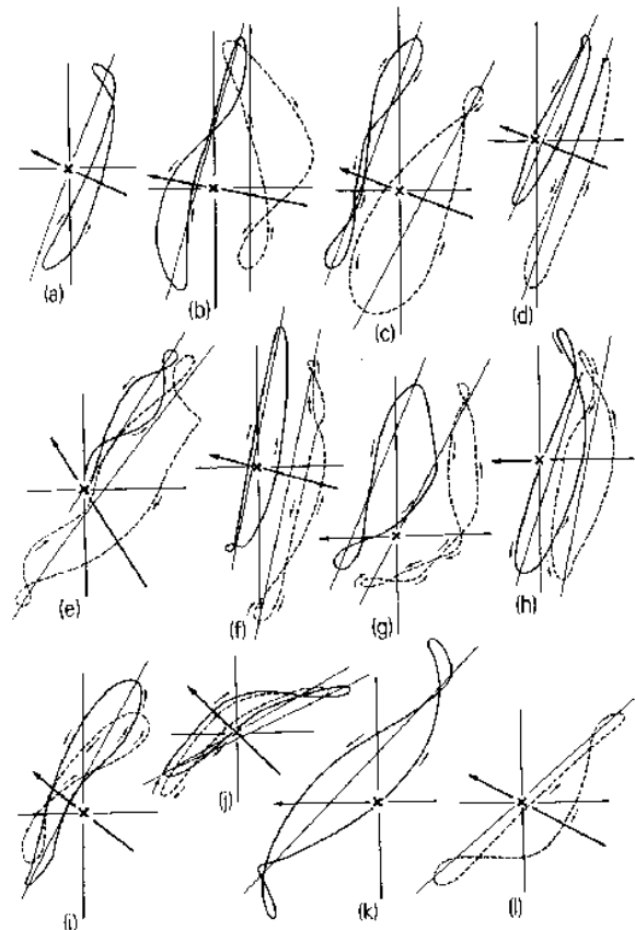
Fig. 5. Wingtip trajectories
