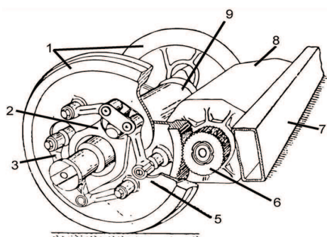
Rys.1. Schemat układu napędowego stosowanego w pojazdach trakcyjnych
