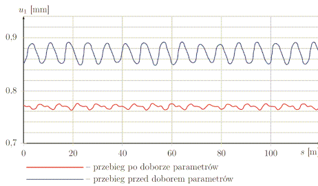
Rys. 6: Zmiana odkształcenia promieniowego przegubu C_5 na drodze 120 m dla parametrów wyjściowych oraz najlepszego otrzymanego zestawu parametrów
