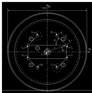
Rys.2. Schemat sprzęgła przyjętego do analizy w układzie koła zestawu
