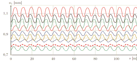
Rys. 4: Zmiana odkształcenia promieniowego przegubu C 5 dla wybranych zestawów parametrów na drodze 120 m
