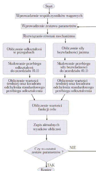
Rys. 3: Schemat algorytmu obliczania wartości funkcji celu dla sprzęgła typu Alsthom
