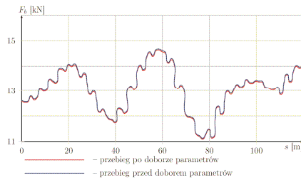
Rys. 7: Zmiana siły bezwładności działającej na jarzmo dla parametrów wyjściowych oraz najlepszego otrzymanego zestawu parametrów
