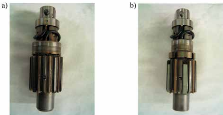
Rys.1. Głowica do honowania podstawowego z płytkami diamentowymi i głowica do honowania wykańczającego płytkami diamentowymi i ceramicznymi
