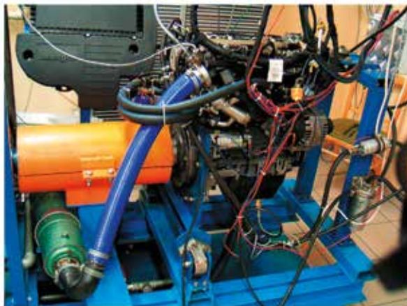
Rys.7. Silnik zamontowany na stanowisku hamulcowym
