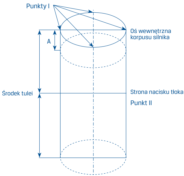
Rys. 6. Miejsca pomiaru chropowatości na tulei cylindrowej
