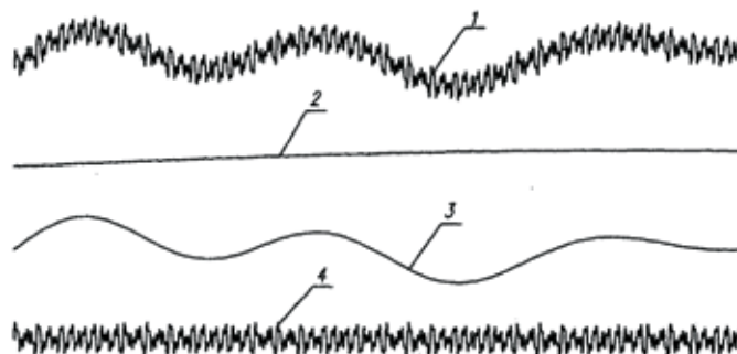
Rys.5. Podział profilu powierzchni (1) na profil kształtu (2), falistości (3) i chropowatości (4)
