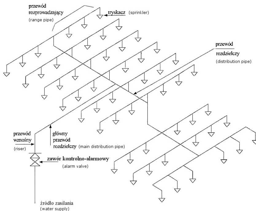
Ryc. 1. Schemat instalacji tryskaczowej [2]
