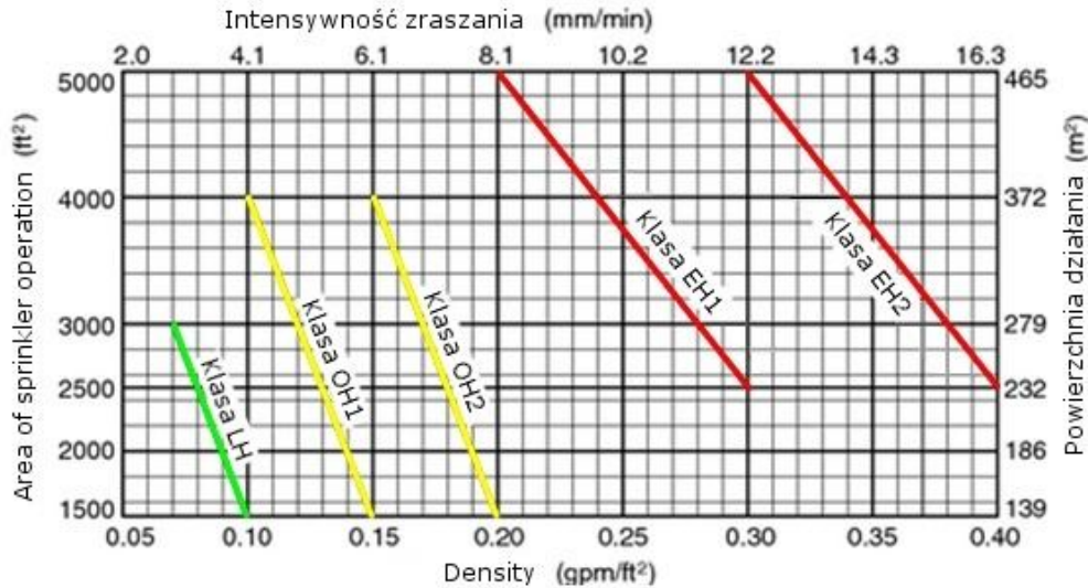
Ryc. 2. Wykres intensywności zraszania i powierzchni zraszania - NFPA 13 [3]
