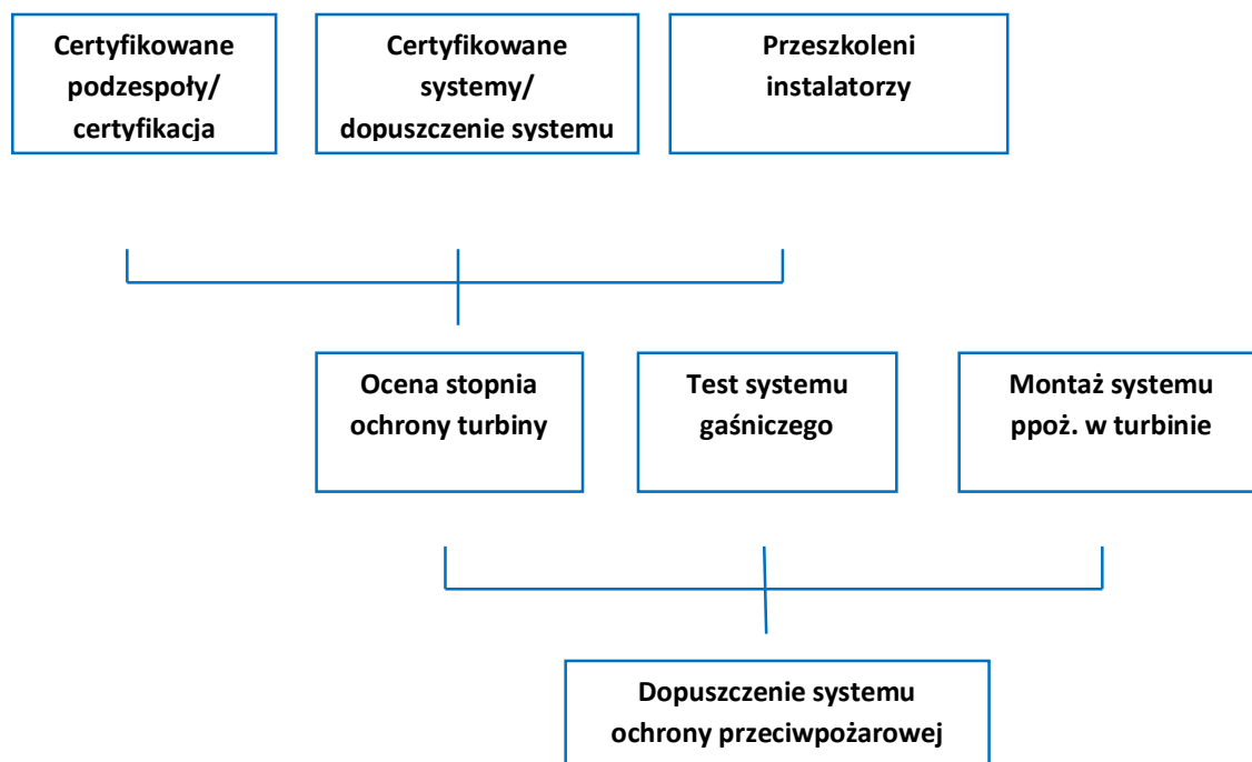
Ryc. 3 Schemat certyfikacji systemu ochrony przeciwpożarowej [7]
