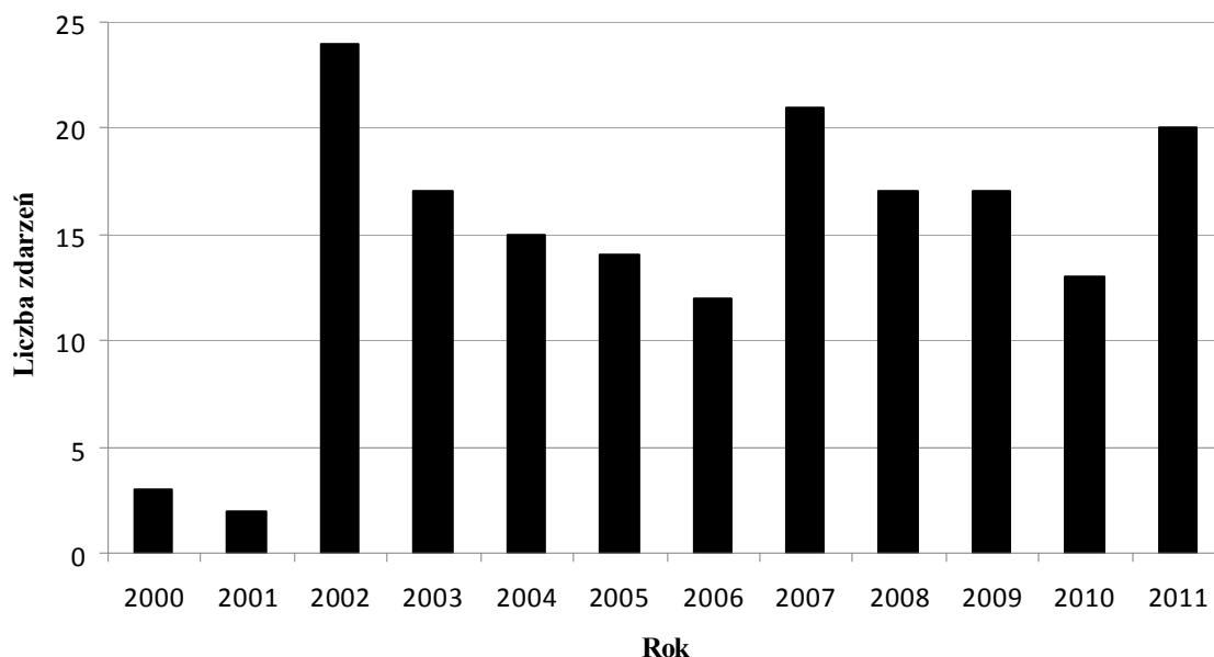
Ryc. 3 Liczba pożarów turbin wiatrowych w latach 2000-2011
