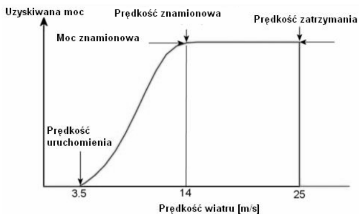
Ryc. 2 Profil mocy turbiny wiatrowej
