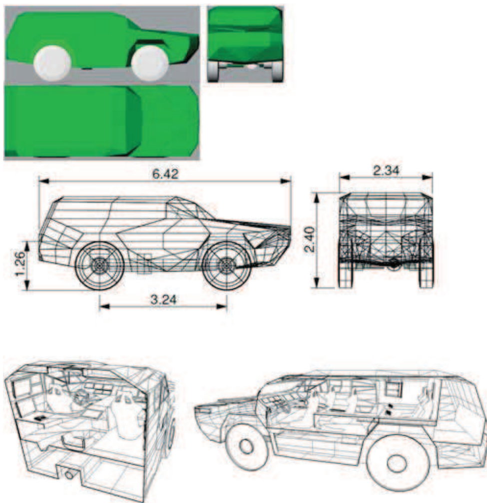
Rys. 1 Widok ogólny, przekrój bryły pojazdu i jej gabaryty (wymiały w metrach) [2][3][4]
