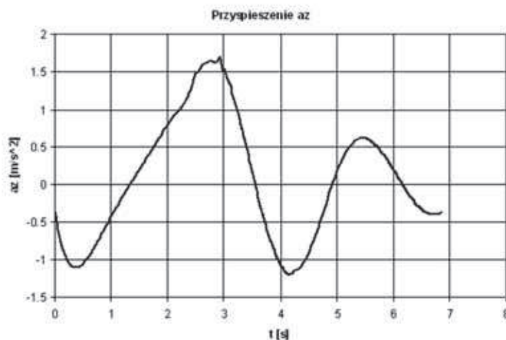
Rys. 8. Przyspieszenie a_z środka masy w funkcji czasu – kąt 20^\circ , prędkość 1\text{m/s} [1][4]
