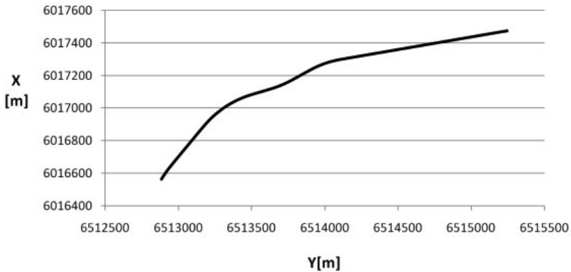
Rys. 1. Przykładowy fragment trasy kolejowej w układzie państwowym „2000”
