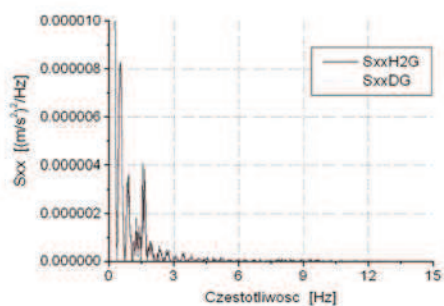
Rys. 14. Fotelik FX, przejazd po nawierzchni asfaltowej, porównanie H2G z DG.
