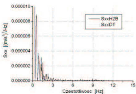
Rys. 13. Fotelik FX, przejazd po nawierzchni asfaltowej, porównanie H2B z DT.
