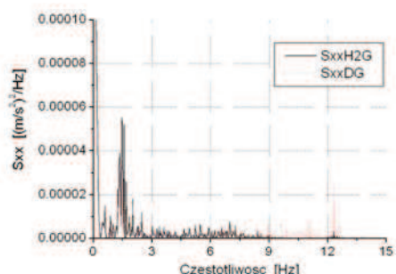
Rys. 16. Fotelik FX, przejazd po nawierzchni nierównej, porównanie H2G z DG.
