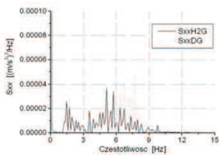
Rys. 12. Fotelik FS, przejazd przez garb, porównanie H2G z DG.
