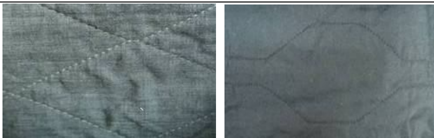
Fot. 2. i 3. Wzory pikowania podszewki z włókniną termoizolacyjną (źródło: zbiór fotografii Zespołu Laboratoriów BS CNBOP)
