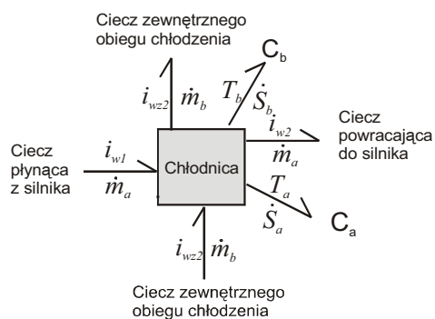
Rys. 7. Ogólny model chłodnicy cieczy do silnika spalinowego [6]. Fig. 7. The basic model of a heat exchanger for a combustion engine [6].
