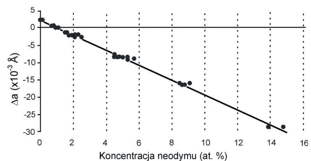
Rys. 5. Wartość \Delta a^+ w zależności od koncentracji jonów Nd^{3+} w warstwie epitaksjalnej Nd: YAG [13].
