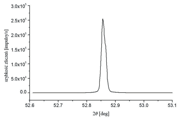
Rys. 10. Dyfraktogram dopasowanej sieciowo struktury Y_{2,97-y}Nd_{0,03}Lu_yAl_{5-z}Ga_zO_{12}/YAG .
