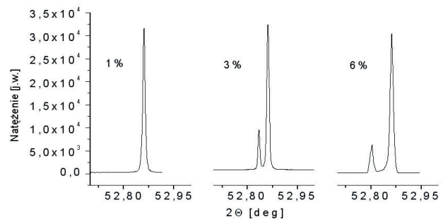
Rys. 4. Dyfraktogramy struktur Nd: YAG/YAG z różnymi koncentracjami jonów Nd^{3+} w warstwie epitaksjalnej.
