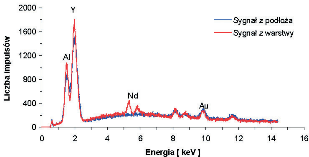
Rys. 1. Widmo fluorescencji rentgenowskiej struktury Nd: YAG/YAG. Pomiar przeprowadzono na szlifie z napyłoną warstwą Au prostopadłym do powierzchni płytki. Fig. 1. X-ray fluorescence spectrum of the Nd: YAG/ YAG epitaxial structure. The measurement was performed on the edge of the structure perpendicular to its surface, with an Au deposited layer.
