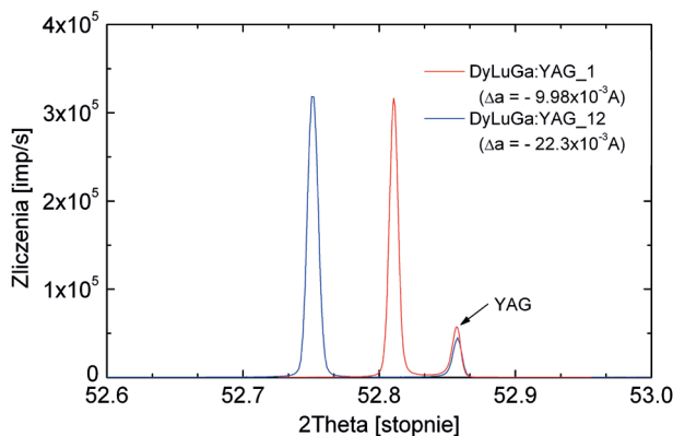
Rys. 14. Dyfraktogramy struktur Y_{3-x-y}Dy_xLu_yAl_{5-z}Ga_zO_{12}/YAG otrzymanych ze składów, w których ułamek molowy Dy_2O_3 wynosi 1,1 \times 10^{-5} i 9,9 \times 10^{-4} .
