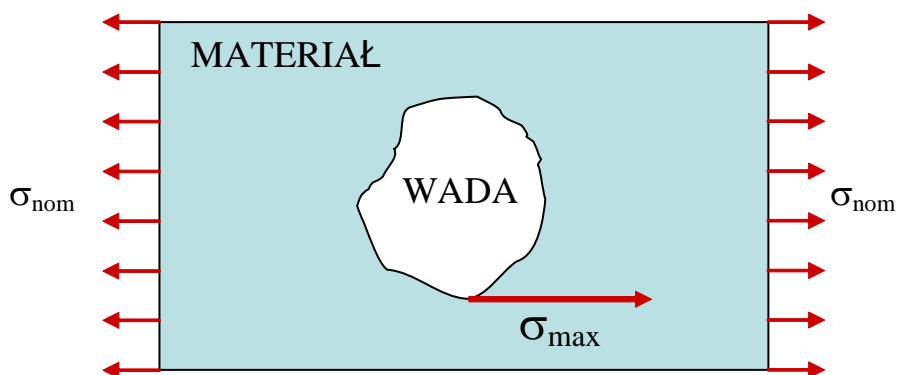
Rys. 1. Wada jako pustka w paśmie rozciągany naprężeniem nominalnym \sigma_{\text{nom}}
