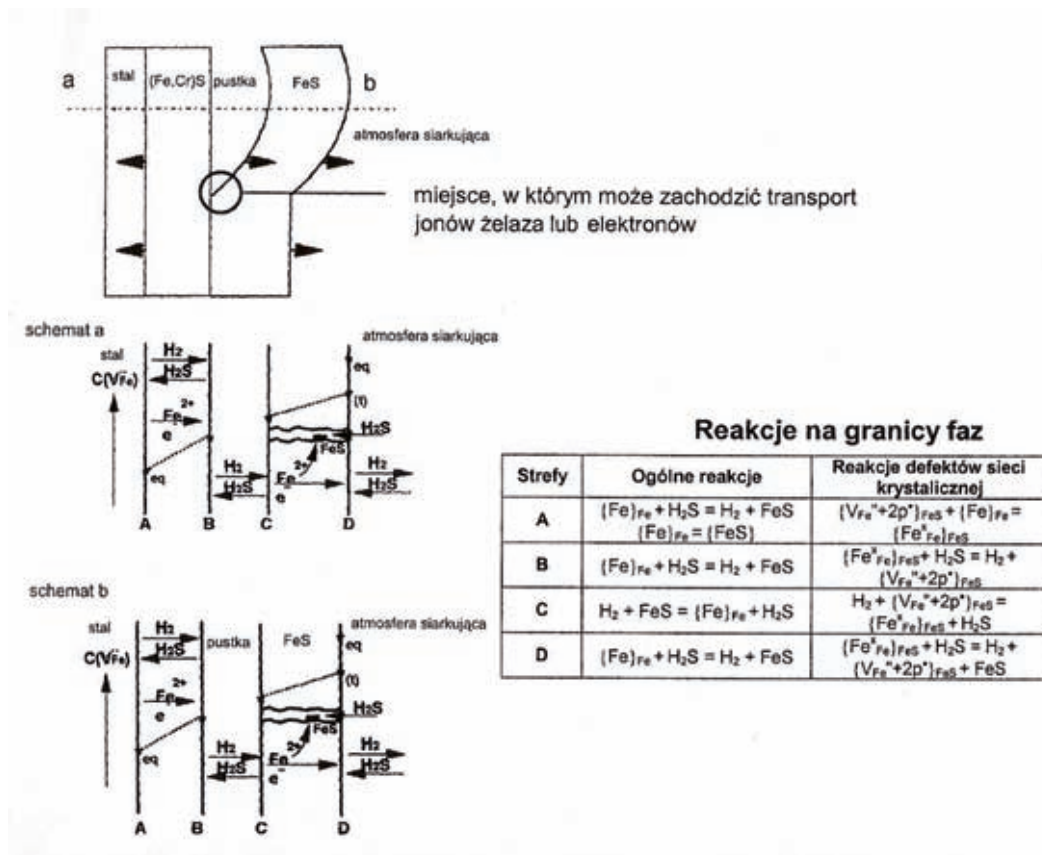
Rys. 9. Schemat procesu transportu, gradientów stężenia oraz reakcje na granicy fazowej, zachodzące w zgorzelinie oraz w miejscu oddzielenia warstwy od podłoża z utworzeniem pustki, według M. Schulte i in. [12]
