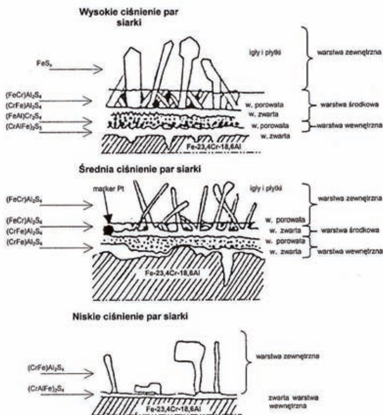
Rys. 5. Schemat budowy wielowarstwowej zgorzeliny na stali FeCr23,4Al18,6 w atmosferze H_2/H_2S w warunkach wysokiego, średniego i niskiego ciśnienia par siarki, według T. Narity i in. [16, 17]
