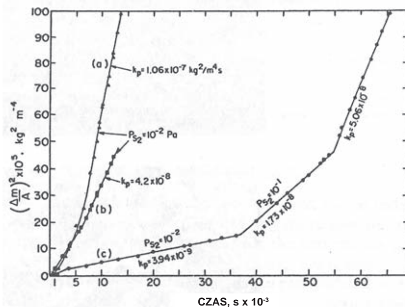
Rys. 10. Wykres parabolicznych przebiegów siarkowania stali FeCr23,4Al18,6 pokrytego warstwą Al_2O_3 a następnie siarkowanego w temperaturze 800^\circ C w atmosferze par siarki ( p_{S_2} = 10^{-2} i 10^{-1} Pa), według T. Narity i in. [16]:
