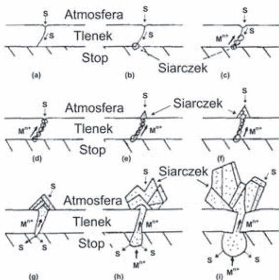
Rys. 11. Schemat mechanizmu odpowiedzialnego za tworzenie się produktów siarkowania na preoksydowanej stali typu Fe-Cr-Al, według S. Mroweca [19]
