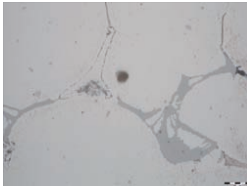
Rys. 19. Mikrostruktura odlewu próbnego w obszarze Al_1. Zgląd trawiony 1% HF, pow. 500x
