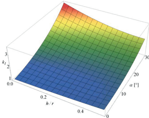
Fig. 10. Relation between \alpha , h/r and coefficient k_{\ell} Rys. 10. Zależność pomiędzy \alpha , h/r i współczynnikiem k_{\ell}
