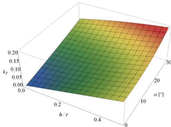
Fig. 11. Relation between \alpha , h/r and coefficient k_p Rys. 11. Zależność pomiędzy \alpha , h/r i współczynnikiem k_p
