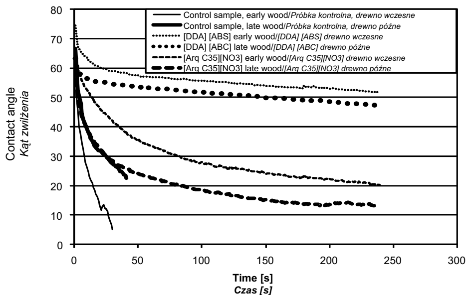
Fig. 2. Contact angles determined on the tangent section of the control samples and the samples treated with [DDA][ABS] and [ArqC35][NO 3 ] Rys. 2. Kąty zwilżenia wyznaczone na przekroju stycznym dla próbki kontrolnej oraz dla próbek zabezpieczonych [DDA][ABS] i [ArqC35][NO 3 ]
