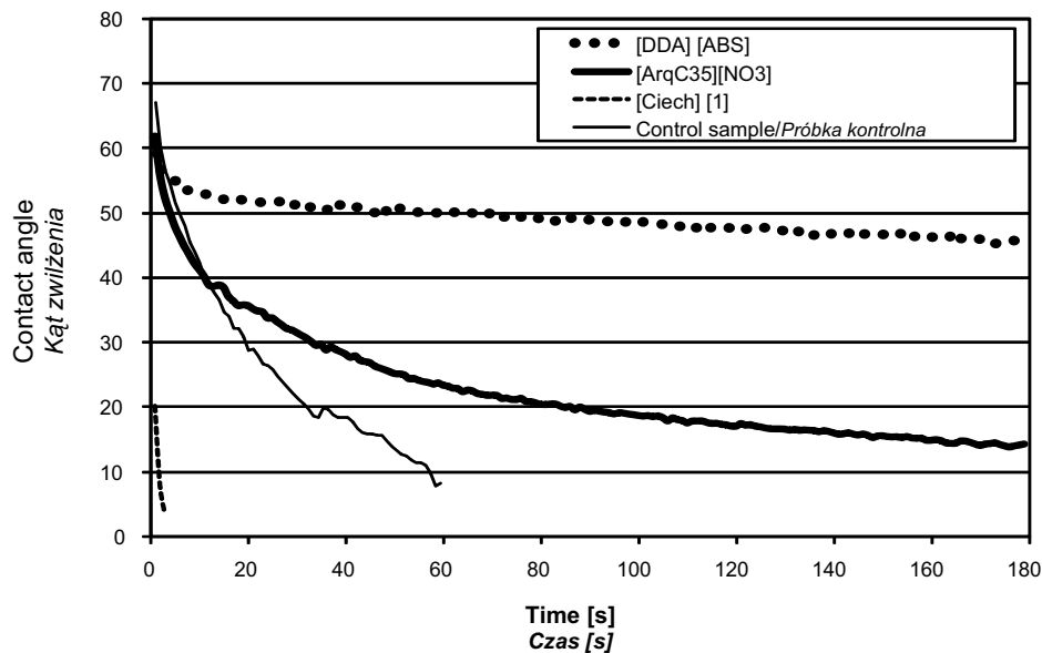
Fig. 1. Contact angles determined on the wood radial section Rys. 1. Kąty zwilżenia wyznaczone na przekroju promieniowym
