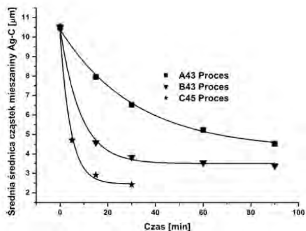
Rys. 6. Zmiany wielkości cząstek mieszaniny Ag-C3 w funkcji czasu mielenia dla wybranych procesów A, B i C.
