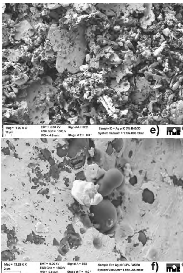
Rys. 9. Obrazy SEM: a) i b) struktury kompozytowe kulistych proszków Ag-C0,1 bezpośrednio po procesie typu C45 mechanicznej syntezy; c) i d) struktury kompozytowe kulistych proszków Ag-C3 po procesie typu C45 mechanicznej syntezy i odmyciu nadmiarowego, swobodnego węgla. e) i f) struktury kompozytowe Ag-C3 płatkowego proszku Ag i kulistego C, bezpośrednio po MS prowadzonej w warunkach procesu C45.
