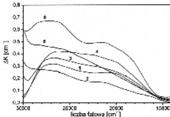
Rys. 15. Widma AA kryształów LN ( D = 1,5 \cdot 10^6\text{ Gy} ) (1); LN:Nd,Mg ( D = 1,5 \cdot 10^6\text{ Gy} ) (2); LN:Tm ( D = 1,5 \cdot 10^6\text{ Gy} ) (3); LN:Yb ( D = 10^6\text{ Gy} ) (4); LN:Er ( D = 1,5 \cdot 10^6\text{ Gy} ) (5); LN:Dy ( D = 10^6\text{ Gy} ) (6).
