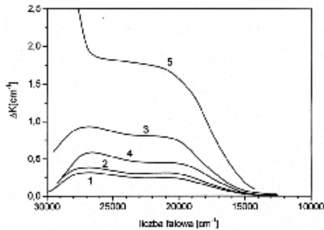
Rys. 20. AA kryształów LN napromieniowanych kwantami gamma: (1) D = 10^6 \text{ Gy} ; elektronami; (2) E = 1.3 \text{ MeV} , D = 10^6 \text{ Gy} ; (3) E = 3.5 \text{ MeV} , D = 10^6 \text{ Gy} lub neutronami; (4) F = 10^{16} \text{ cm}^{-2} ; (5) F = 10^{18} \text{ cm}^{-2} [80].
