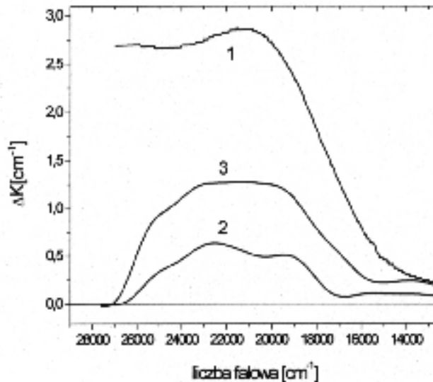
Rys. 16. Widma AA kryształów: LN:Fe (0,2%) napromieniowanych kwantami gamma ( E = 1,25 \text{ MeV} , D = 10^6 \text{ Gy} ) (1) oraz LN:Fe (0,03%) napromieniowanych kwantami gamma ( E = 1,1 \text{ MeV} , D = 8 \times 10^5 \text{ Gy} ) (2) [80]; elektronami ( E = 3,5 \text{ MeV} , F = 10^{16} \text{ cm}^{-2} ) (3) [80].
