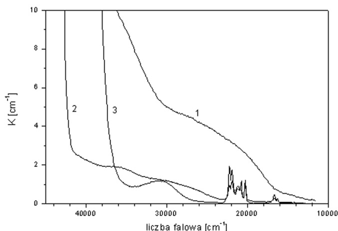
Rys. 9. Widma absorpcji kryształów: YAP (1); YAP:Pr (2); oraz YAP:Pr,Ca (3).
