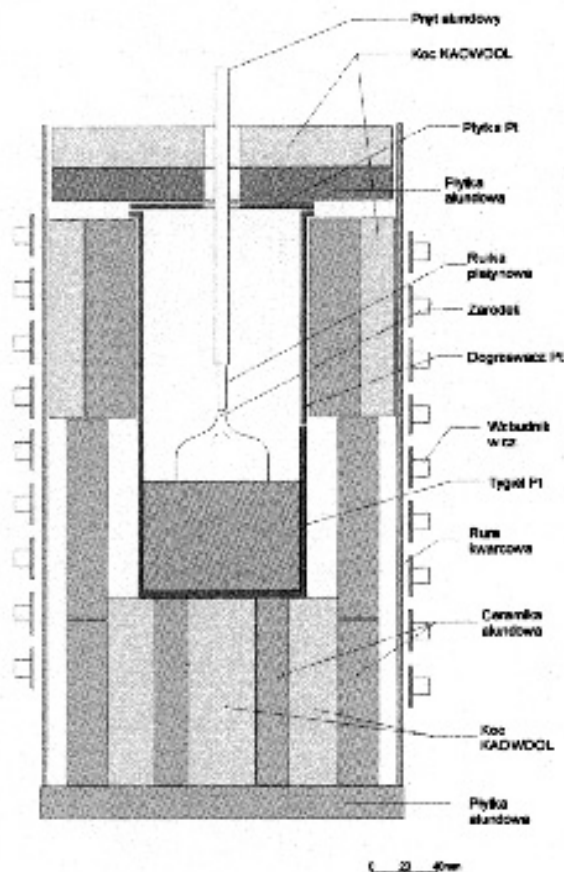
Rys. 6. Schemat cieplnego układu wzrostu kryształów \text{LiNbO}_3 .
