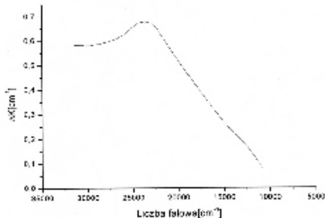
Rys. 21. Widmo niestabilnej AA kryształu YAP:Pr.
