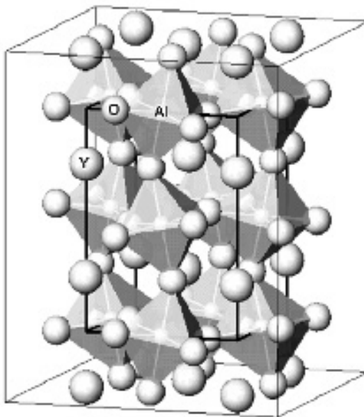
Rys. 1. Struktura kryształu \text{YAlO}_3 [50]. Fig. 1. Crystal structure of \text{YAlO}_3 [50].
