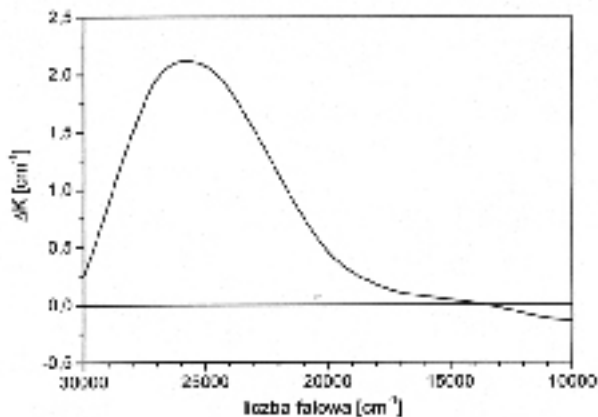
Rys. 17. AA kryształu LN:Cu (0,03%) napromieniowanego kwantami gamma ( D = 10^5 \text{ Gy} ). Fig. 17. AA spectra in LN:Cu (0,03%) crystal gamma quantum irradiated ( D = 10^5 \text{ Gy} ).
