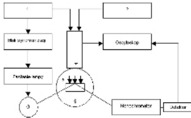
Rys. 8. Schemat stanowiska do pomiaru niestabilnej AA indukowanej przez impulsy elektronów: 1 - wyzwalacz impulsów elektronowych; 2 - generator wysokiego napięcia; 3 - lampa KKSSZ-500; 4 - generator impulsów elektronowych; 5 - komora pomiarowa.
