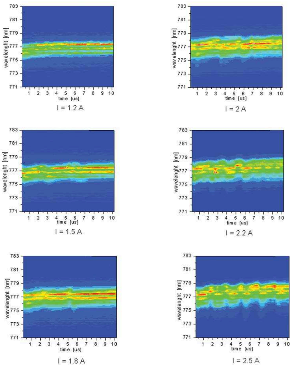
Rys. 9. Seria charakterystyk spektralnych z „zagęszczonym” próbkowaniem (odstęp pomiędzy kolejnymi próbkami: 250 ns) dla diody z heterostruktury asymetrycznej.
