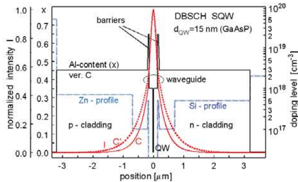
Rys. 1. Schemat heterostruktury symetrycznej DBSCH-SQW dla diod laserowych dużej mocy. Linia czarna – profil składu (Al-content), linie niebieskie - profile domieszkowania Zn i Si; linie czerwone - obliczone rozkłady pola optycznego dla dwóch wersji projektowych (wersje C i C'). Profil składu (Al-content) podany tylko dla wersji C.
