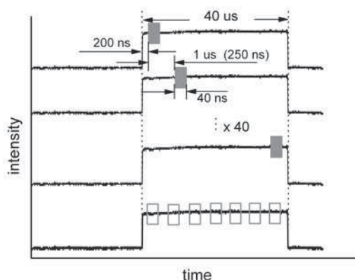
Rys. 4. Sposób wykonywania pomiarów spektralnych z rozdzielczością czasową przy pomocy kamery ICCD. Na tle impulsów optycznych rejestrowanych fotodiodą (zatem scałkowanych po całym widmie promieniowania) zilustrowano sekwencję czasową próbkowania w tej pracy.
