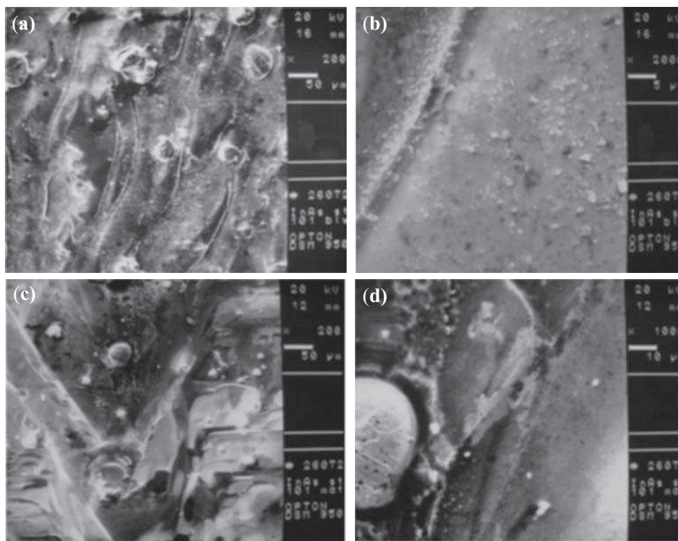
Rys. 6. Obrazy morfologii po procesie monokryształizacji ścianek na stożkowej części monokryształu InAs: a, b) ścianka błyszcząca; c, d) ścianka matowa.
