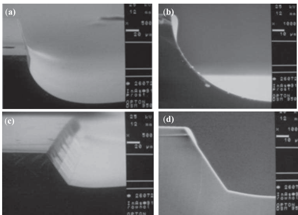
Rys. 4. Obraz profilu wytrawienia przy krawędzi maski tlenkowej na przełomie płytki InAs: a), b) przełom prostopadły do głównego ścieżca bazowego wg standardu SWMI ( dovetail-groove ”; c), d) przełom równoległy do głównego ścieżca bazowego wg standardu SEMI - V-groove ”.
