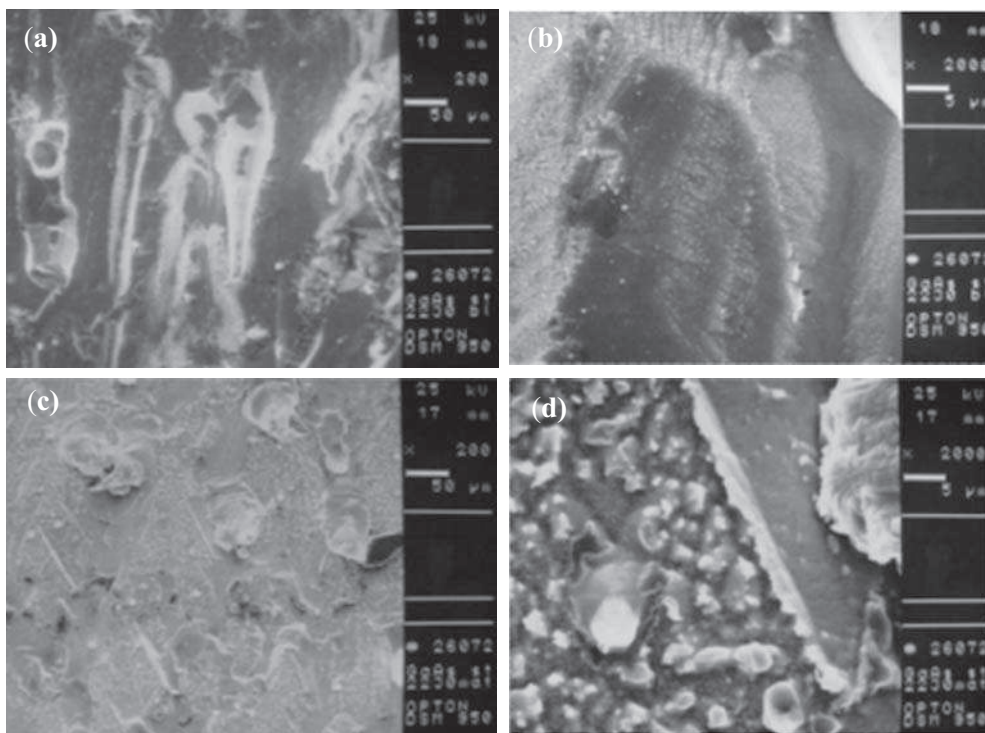
Rys. 5. Skaningowe (SEM) obrazy morfologii, po procesie monokrystalizacji ścianek na stożkowej części monokryształu GaAs: a), b) ścianka błyszcząca; c), d) ścianka matowa.
