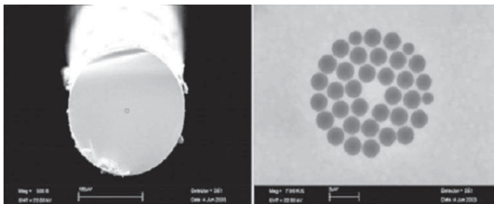
Rys. 1. Pierwszy światłowód całoszklany SOHO [4].
