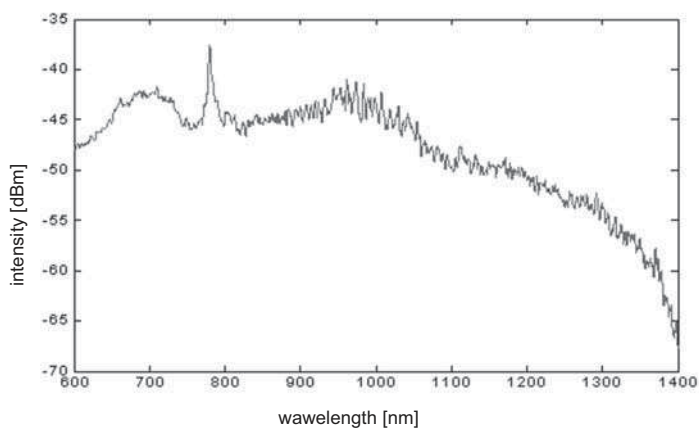
Rys. 12. Spektralny zakres pracy źródła superkontinuum użytego w eksperymencie. Fig. 12. Spectrum of nonlinear PCF based supercontinuum light source used in the experiment.
