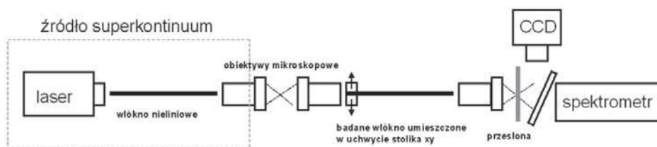
Rys. 11. Użyte stanowisko pomiarowe.
