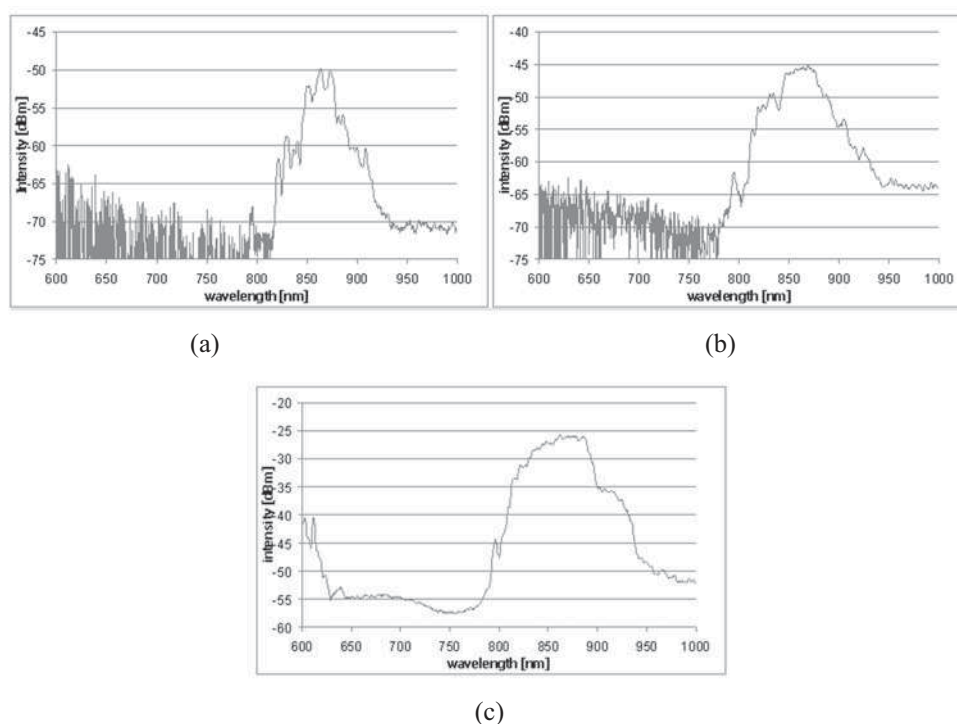
Rys. 14. Zarejestrowany zakres spektralny transmisji dla dwuszklanego włókna pobudzanego białym światłem pochodzącym ze źródła superkontinuum dla próbek o długości: a) 80,6 cm; b) 55,8 cm; c) 24,1 cm.
