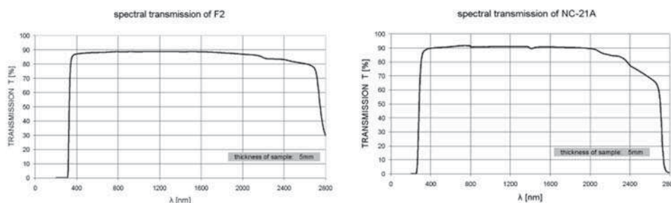
Rys. 5. Transmisja spektralna szkieł F2 i NC-21.
