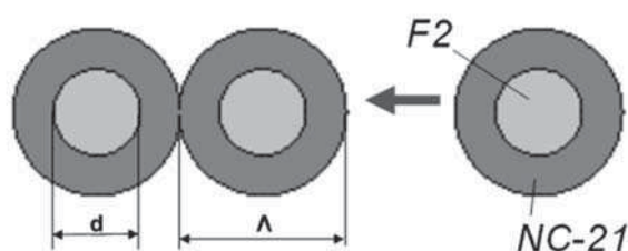
Rys. 4. Metoda układania makrostruktury dla sieci kryształy fotonicznego o parametrach d i d/\Lambda na przykładzie dwuszkłanych prętów wykonanych ze szkła F2 i NC-21.
