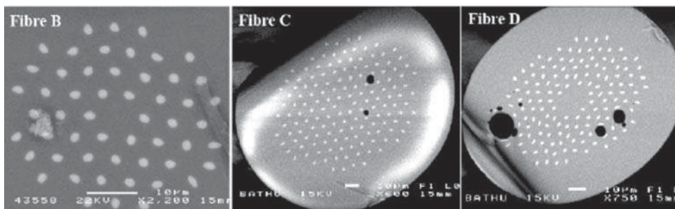
Rys. 2. Zdjęcia z mikroskopu elektronowego próbek całoszklanych włókien fotonicznych z widocznymi deformacjami struktury [7].
