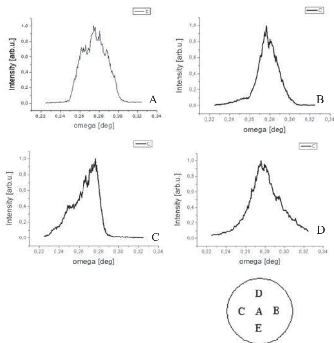
Rys. 13. Rentgenowskie krzywe reflektometryczne otrzymane w ustawieniu non-specular dla różnych miejsc na próbce nr 7 – Si(111) o grubości 80 \mu\text{m} obustronnie polerowanej („S16_31”). Miejsca pomiarowe schematycznie pokazują litery A-D.
