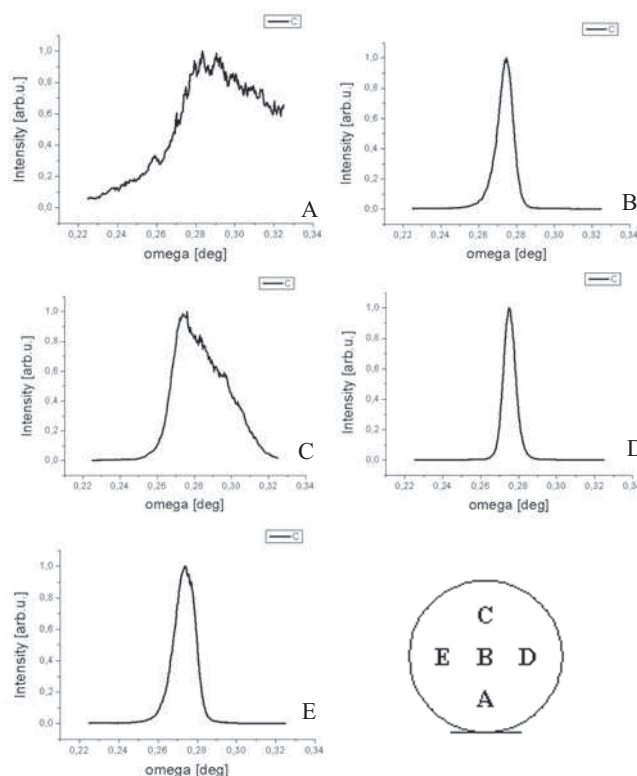
Rys. 14. Rentgenowskie krzywe reflektometryczne otrzymane w ustawieniu non-specular dla różnych miejsc na próbce nr 8 – Si(111) o grubości 80 \mu\text{m} obustronnie polerowanej („S16_35”). Miejsca pomiarowe schematycznie pokazują litery A-E.
