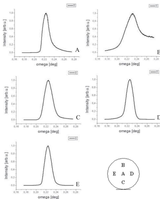
Rys. 10. Rentgenowskie krzywe reflektometryczne otrzymane w ustawieniu non-specular dla różnych miejsc na próbce nr 4 Si(111) o grubości 280 \mu\text{m} z 100 dezorientacją („dez10”). Miejsca pomiarowe schematycznie pokazują litery A-E.
