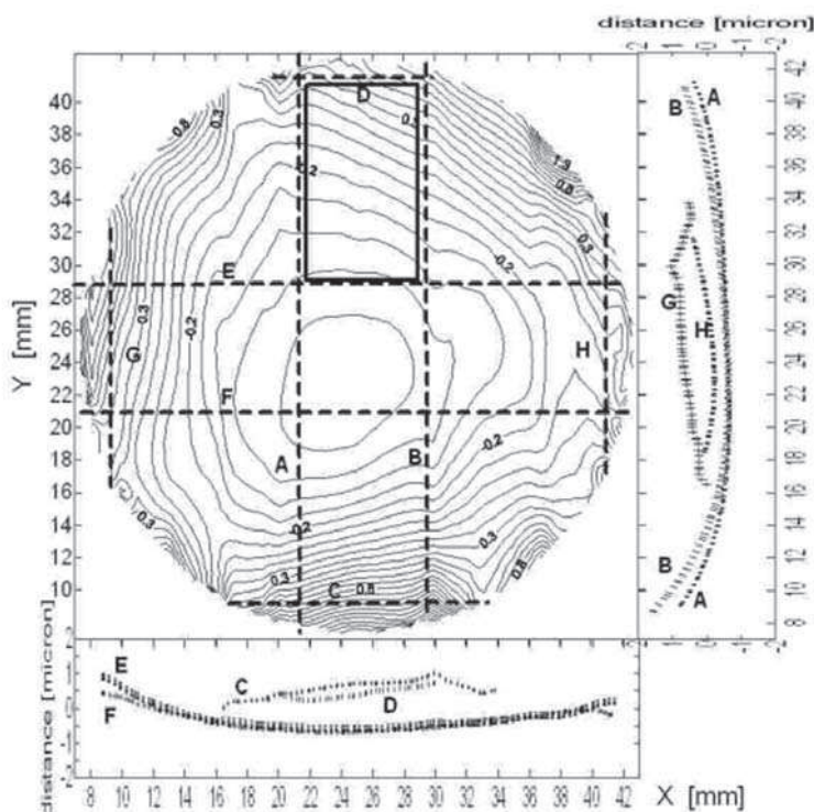
Rys. 14a. Konturowa mapa kształtu powierzchni uzyskana metodą konfokalną z przekrojami w miejscach badanych za pomocą XRR.
