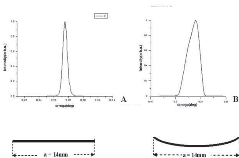
Rys. 5. Przykładowe krzywe dla dwóch próbek: A) z bardzo małym odstępstwem od płaskości, FWHM = 26 sek \Rightarrow h = 0.3 \mu\text{m} , B) ze znacznie większym, FWHM = 85 sek \Rightarrow h = 1.435 \mu\text{m} .
