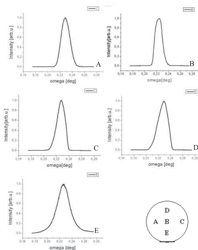
Rys 7. Rentgenowskie krzywe reflektometryczne otrzymane w ustawieniu non-specular dla różnych miejsc na próbce nr 1 – Si(001) o grubości 300 \mu\text{m} („300”). Miejsca pomiarowe schematycznie pokazują litery A-E.
