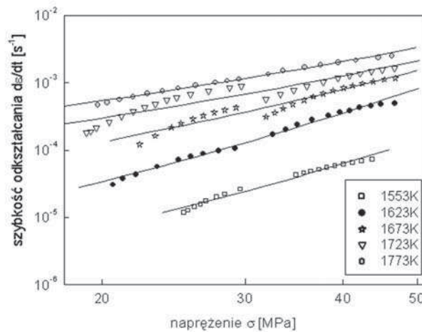
Rys. 2. Szybkość odkształcania nadplastycznego d\epsilon/dt ceramiki cyrkonowej w funkcji przyłożonego naprężenia \sigma dla różnych temperatur. Test wykonano w układzie ściskania.
