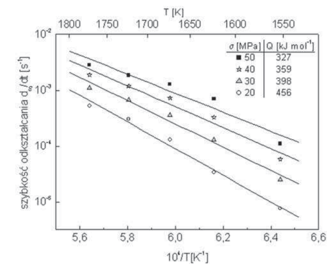
Rys. 3. Szybkość odkształcania nadplastycznego d\varepsilon/dt dla ceramiki cyrkonowej w funkcji odwrotności temperatury dla różnych naprężeń \sigma i wyznaczone stąd energie aktywacji Q .
