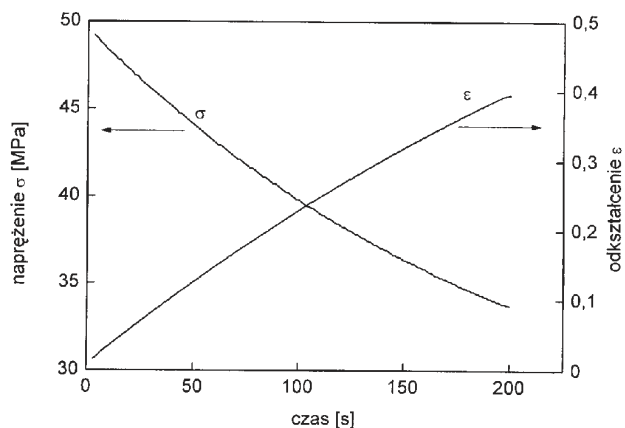
Rys. 1. Odkształcenie \epsilon oraz naprężenie \sigma w funkcji czasu dla próbki z ceramiki cyrkonowej w teście na ściskanie przeprowadzonym w temperaturze 1773 K. Naprężenie początkowe wynosiło 50 MPa.
