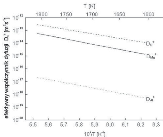
Rys. 9. Temperaturowe zależności efektywnych współczynników dyfuzji jonów Mg^{2+} , Al^{3+} i O^{2-} w spinelu na podstawie odpowiednio [1, 13-14] ( X = Mg, Al lub O ).
