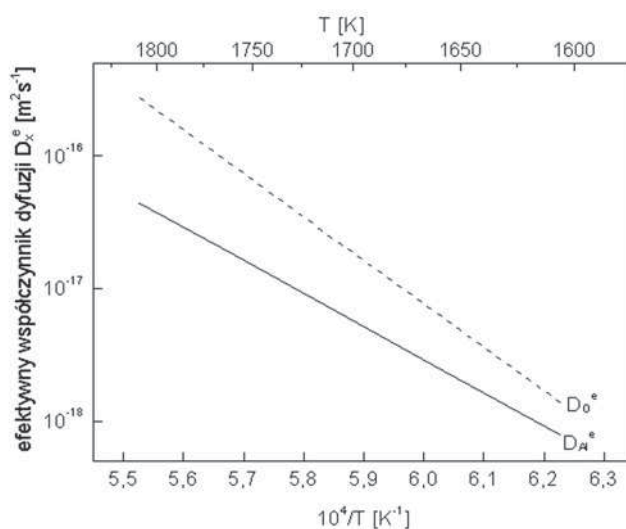
Rys. 7. Temperaturowe zależności efektywnych współczynników dyfuzji jonów \text{Al}^{3+} i \text{O}^{2-} w \text{Al}_2\text{O}_3 na podstawie odpowiednio [11-12] ( X = \text{Al} lub \text{O} ).
