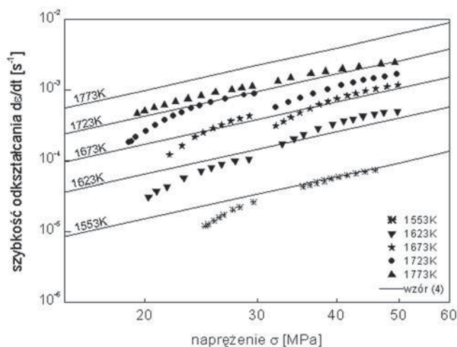
Rys. 6. Dane eksperymentalne z Rys. 2 z naniesionymi krzywymi teoretycznymi obliczonymi z równania (4) (linie ciągłe) dla ceramiki cyrkonowej.
