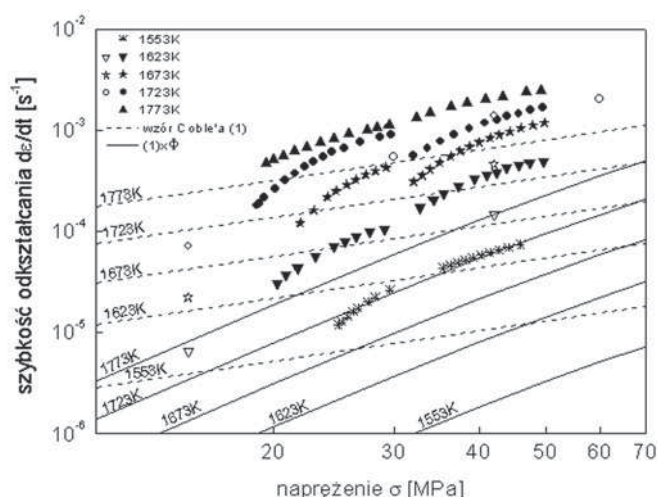
Rys. 5. Dane eksperymentalne z Rys. 2 (zaczernione symbole) z naniesionymi krzywymi teoretycznymi obliczonymi z równania Coble'a (1) (linie przerywane) i dla (1) \times \Phi (linie ciągłe) dla ceramiki cyrkonowej. Dla porównania naniesiono również znormalizowane do wielkości ziarna d = 0.29 \mu\text{m} (przyjmując p = 1.6 [7] gdzie p jest wykładnikiem potęgowym przy wielkości ziarna ((1) z Cz.1)) dane z pracy Owena i Chokshi [8] (puste symbole) dla T = 1623, 1673 i 1723 K dla d = 0.41 \mu\text{m} (normalizacja polegała na pomnożeniu szybkości odkształcania dla d = 0.41 \mu\text{m} przez czynnik (0.41/0.29)^{1.6} = 1.74 ).
