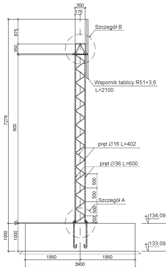
Rys. 3. Boczny rzut bramownicy kratowej (wg proj. P. Łętowskiego)
