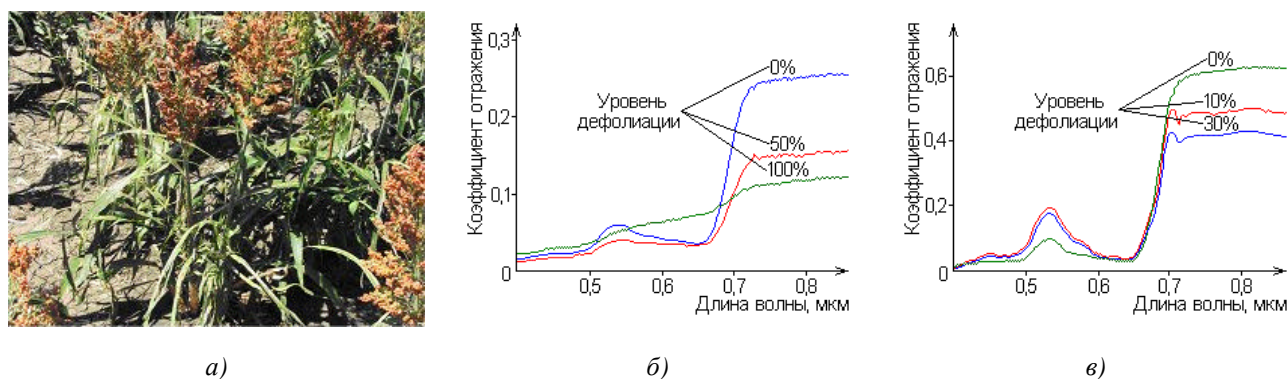
Рис. 3. Дефолиация и ее влияние на спектр сельскохозяйственных культур: а) – поврежденное градом 1 февраля 2004 г. сорго в окрестности г. Долби (Австралия); б) – спектры полога кукурузы (стадия 8-12 листьев); в) – спектры полога сорго (стадия 9 листьев)
