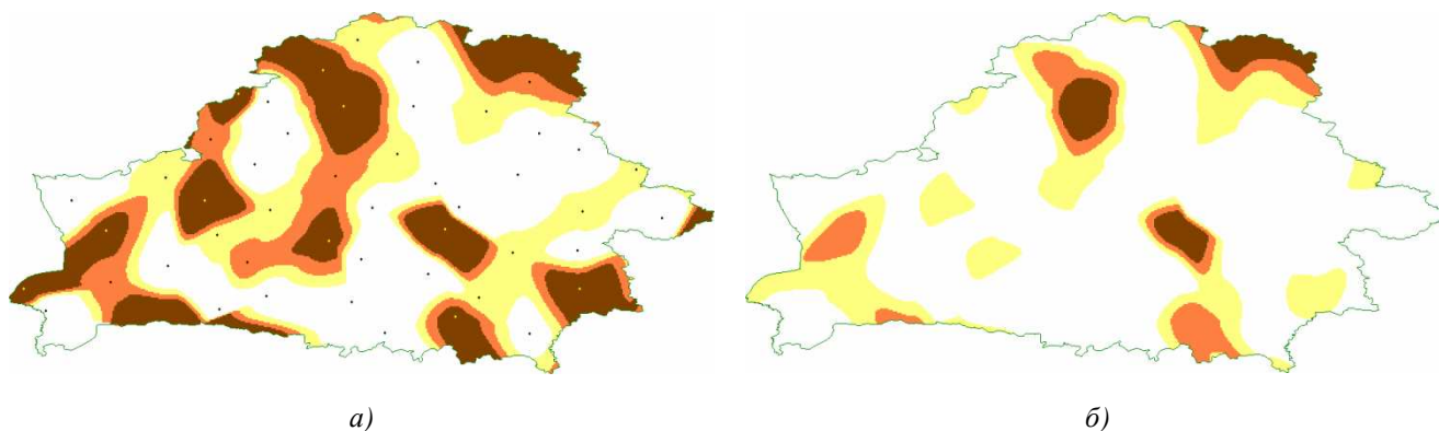
Рис. 2. Оценка риска выпадения града по данным за 2006-2008 гг.: а) – учтены все случаи выпадения града; б) – учтены случаи выпадения града в период с март по октябрь (+ – метеостанции; белый, желтый, оранжевый, коричневый – соответственно до 2, от 2 до 3, от 3 до 4, от 4 и выше случаев выпадения града в течение трех лет)
