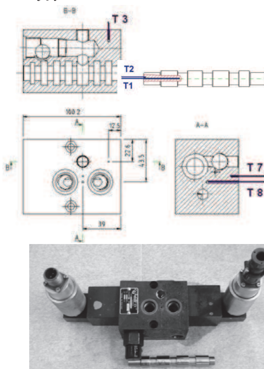
Rys. 3. Rozdzielacz RE2510/101 firmy Hydrotor T1, T2 - termopary umieszczone w suwaku T3, T7, T8 - termopary umieszczone w korpusie
