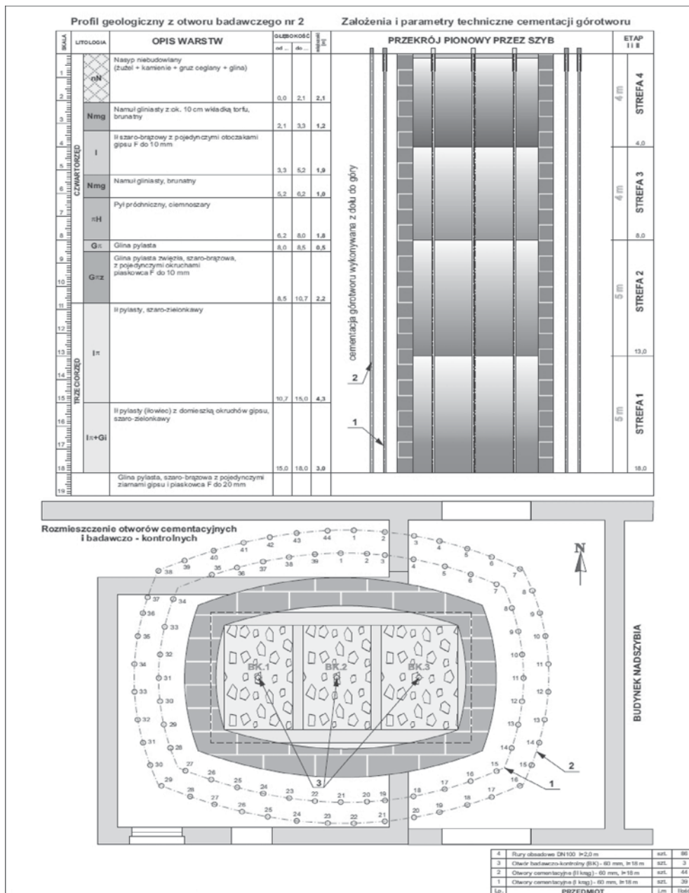
Rys. 2. Strefy doszczelnienia oraz rozmieszczenie otworów cementacyjnych i badawczo-kontrolnych (BK1-BK3) [6]
