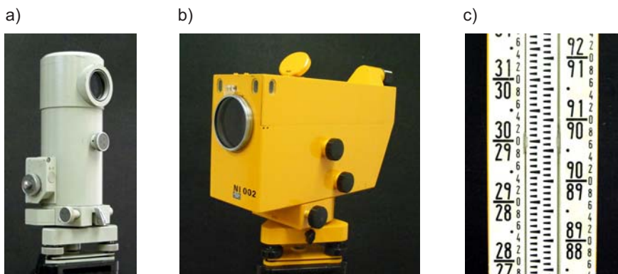
Rys. 1. Niwelatory precyzyjne optyczne: a) Ni 007, b) Ni 002 oraz c) fragment łąty inwarowej
