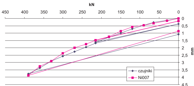
Rys. 6. Wykres z przebiegiem dwóch zgodnych obserwacji
