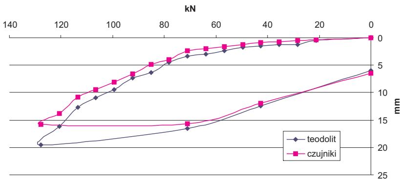
Rys. 9. Wykres z przebiegiem obserwacji przemieszczeń bocznych
