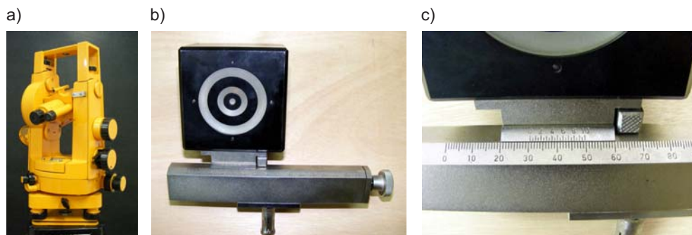
Rys. 4. a) teodolit Theo 010, b) i c) przesuwana tarczka celownicza z podziałką i noniuszem
