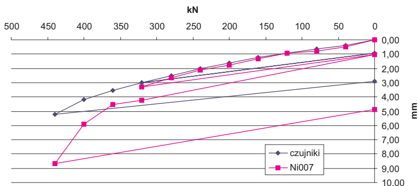
Rys. 7. Wykres z przebiegiem dwóch rozbieżnych obserwacji
