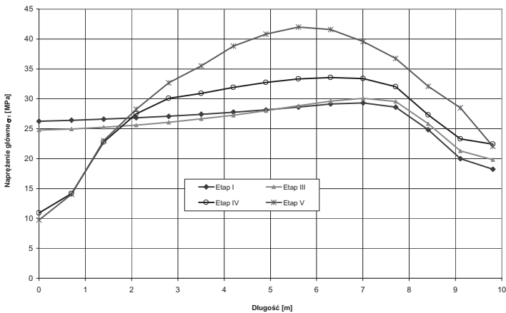
Rys. 7. Rozkład naprężeń głównych \sigma_1 w filarze pomiędzy chodnikiem podścianowym B-11 a chodnikiem wentylacyjnym B-13 przy szerokości filara 8,5 m
