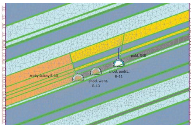
Rys. 2. Sytuacja górniczo-geologiczna wokół chodnika podścianowego B-11
