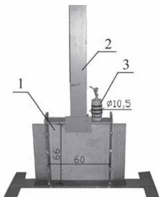
Rys. 3. Stanowisko do badań modelowych
