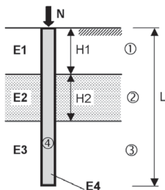
Rys. 1. Pał w trójwarstwowym podłożu gruntowym
