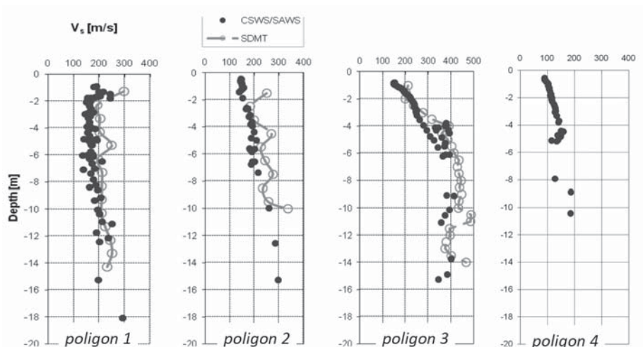
Rys. 2. Wyniki bezpośrednich pomiarów sejsmicznych prędkości fali poprzecznej V_s w funkcji głębokości dla: łąw plicieńskich — poligon 1, piasków rzecznych — poligon 2, glin zwałowych — poligon 3, mad — poligon 4
