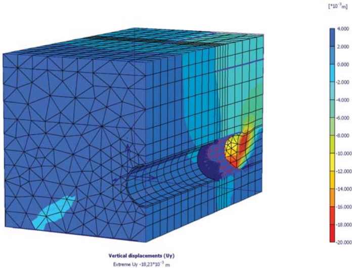
Rys. 4. Siatka elementów obrazująca rozkład pionowych przemieszczeń. Największe przemieszczenie pionowe w rejonie tarczy wynosi 18,23 mm. [11]
