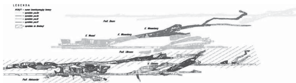
Rys. 4. Schemat przestrzenny rejonu komór Jakubowice [17]
