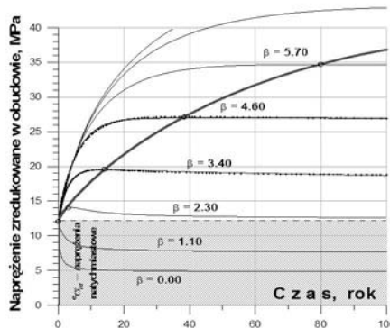
Rys. 9. Zależność maksimum \sigma_{rd} od czasu i podatności obudowy
