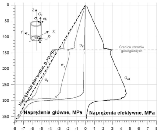
Rys. 4. Przykład rozkładu naprężeń głównych i zredukowanych w szybie bez obudowy
