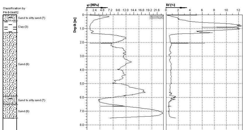
Rys. 6. Profil geologiczny wg klasyfikacji Młynarka i zespołu z 1997 roku
