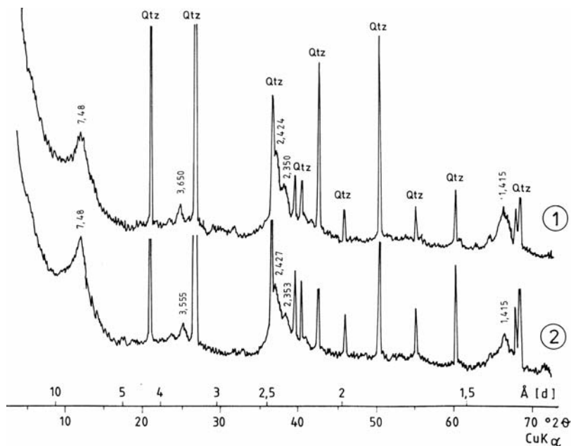
Fig. 6. Dyfraktogramy rentgenowskie tlenków manganu z poliminerальной żyły z diabazu Niedźwiedziej Góry (patrz też tabela 1 – próbki 1 i 2). Qtz – refleksy pochodzące od niedającej się odseparować domieszki kwarcu
