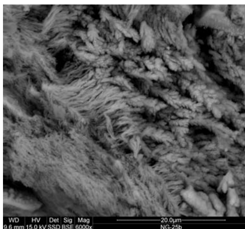
Fig. 5. Dendrytopodobne (prawy fragment fotografii) oraz pierzaste (lewy fragment) skupienia tlenków manganu w poliminerальной żyły z diabazu Niedźwiedziej Góry. SEM
