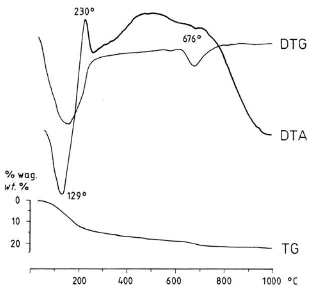
Fig. 8. Krzywe termiczne tlenków manganu z diabazu Niedźwiedziej Góry
