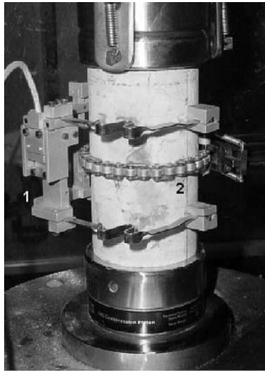
Rys. 5. Próbka skalna z założonymi czujnikami:
