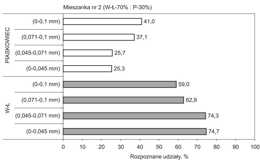
Rys. 6. Porównanie rozpoznanych udziałów dwóch typów rud z rzeczywistymi w mieszankach o przewodze rudy węglanowo-łupkowej dla różnych klas ziarnowych
