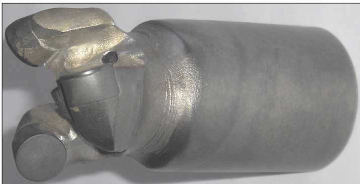
Rys. 1. Świder małosrednicowy PDC używany w wierceniach podziemnych
