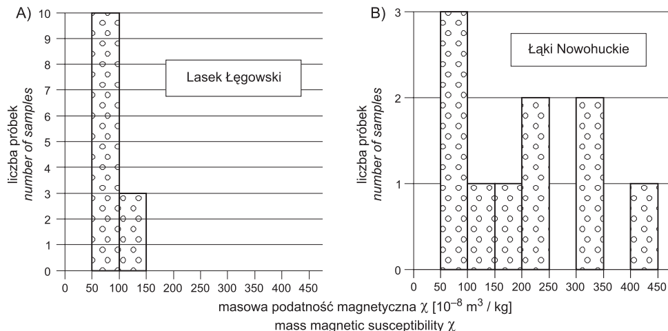
Fig. 5. Histogramy masowej podatności magnetycznej próbek gleb pobranych na terenie: A) Lasku Łęgowskiego; B) Łąk Nowohuckich
