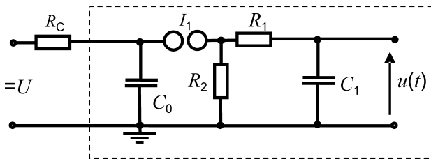
Rys. 5. Podstawowy schemat ideowy jednostopniowego generatora napięć uderowych
