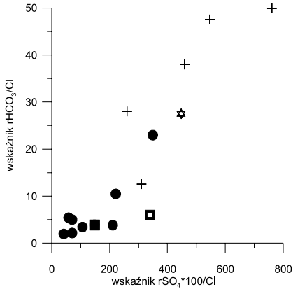
Rys. 1. Zależność między wskaźnikami hydrochemicznymi w badanych wodach
